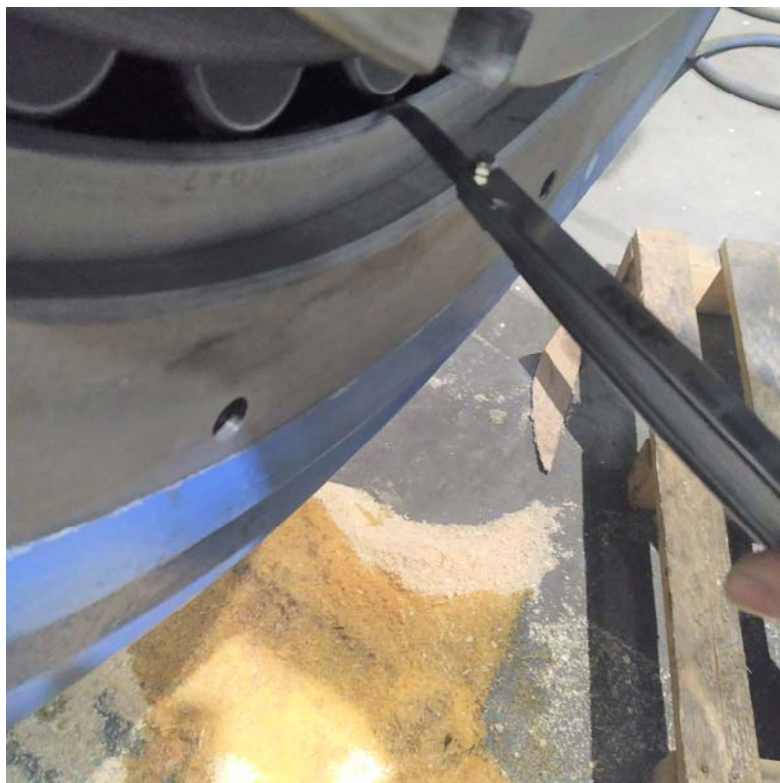
Galgado de juego radial según norma de rodamiento
